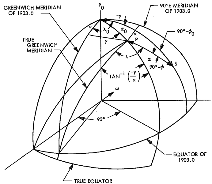
Fig. 4. Latitude and longitude relative to mean pole of 1903.0 and true pole of date
